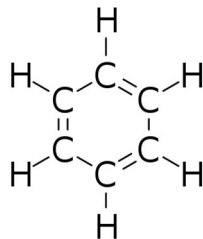
Rysunek 12. Struktura cząsteczki benzenu 7
