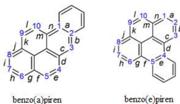
Rysunek 13. Porównanie cząsteczki benzo(a)pirenu oraz benzo(e)pirenu 8
